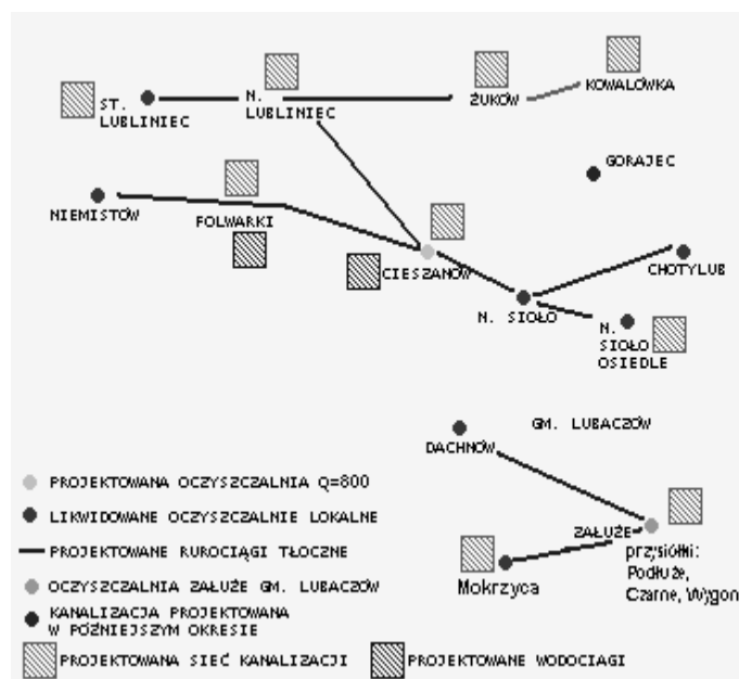
Rysunek 1 Schemat projektowanego systemu gospodarki kanalizacyjnej w Gminie Cieszanów i Lubaczów
