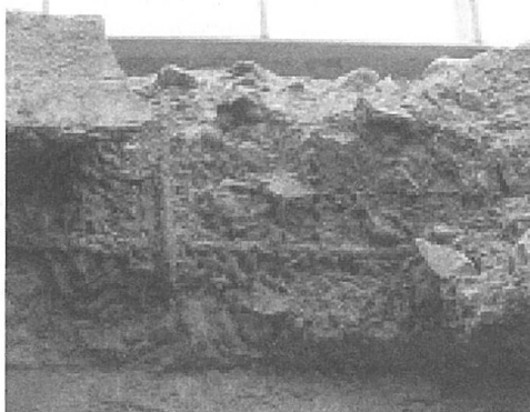
Foto 8- widoczne odsłonięte zbrojenie. od strony Sanu,
