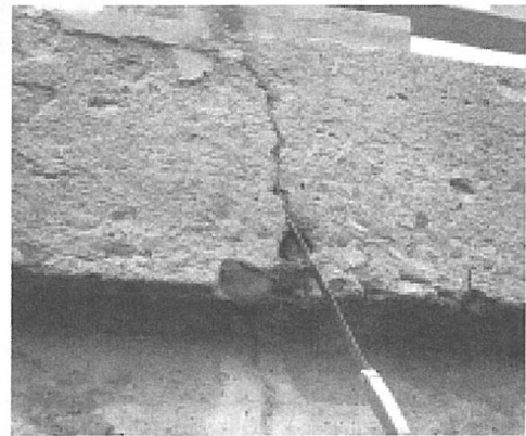
Foto 6- w szparę pęknięcia został włożony przecinak do kopert.
