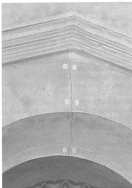
powiększenie muru nad oknem, z naklejonymi na szparę pęknięcia (w pionie i wewnątrz) 3 wskaźników-taśm, przy pomocy 6 krążków, pęknięcie na 1.11.2016 r miało ok. 2 mm, a obecnie ma już 4 mm! co każdy z Czytelników Kresowiaka może sprawdzić
