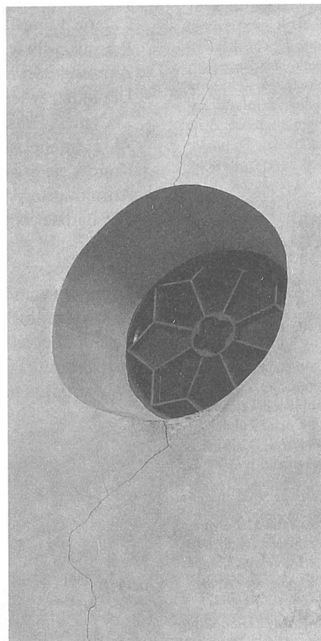
Kaplica ściana północna, pęknięcia widoczne: nad, wewnątrz i pod oknem, powiększające się.
